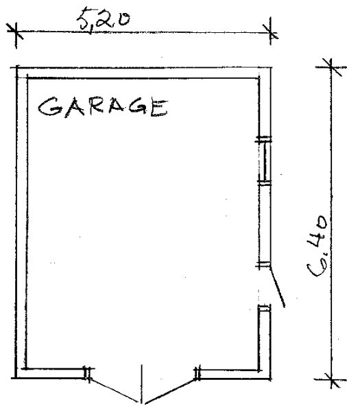
PLAN 1:100
